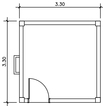
PLANTA BAIXA DO PAVIMENTO FUNDAÇÃO escala.....1:75
