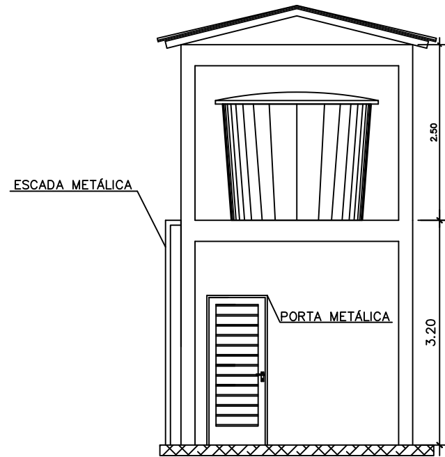
FACHADA FRONTAL escala.....1:75
